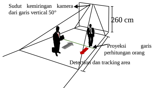
Gambar 7: Skema pemasangan kamera dan pengambilan data uji
