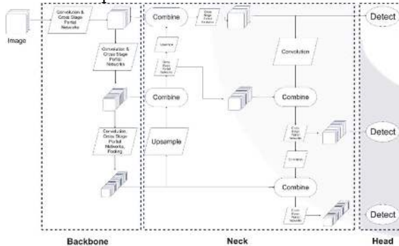
GAMBAR 3 (C) Arsitektur YOLOv8.
