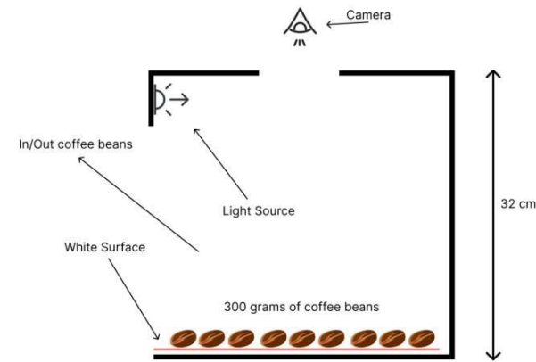
GAMBAR 6 (F) Ilustrasi akuisisi citra dari 300 gram biji kopi hijau Arabika Mandheling.
