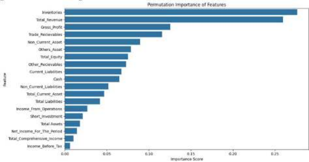
GAMBAR 4.11. Grafik Hasil Urutan Fitur Yang Paling Berpengaruh Untuk Model XGBoost
