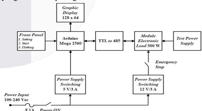
GAMBAR 4 (BLOK DIAGRAM KESELURUHAN SISTEM)
