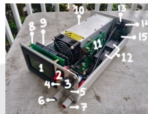
a) Tampak Atas Terbuka
