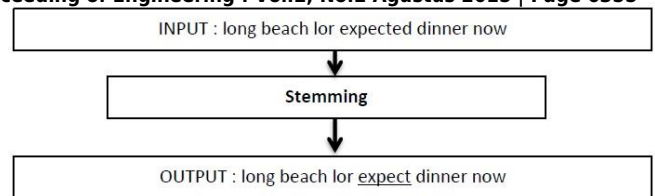
Gambar 5 : Proses Stemming
