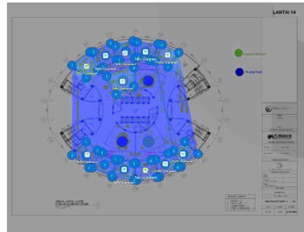
GAMBAR 14 Heatmap Signal to Interference Ratio Pada Lantai 14
