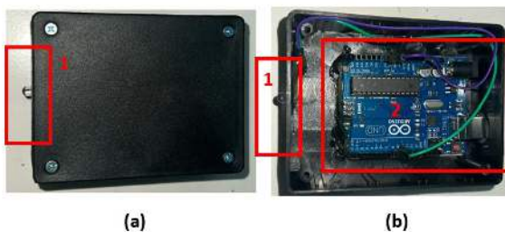
GAMBAR 6 HASIL PERANCANGAN TRANSMITTER LI-FI
