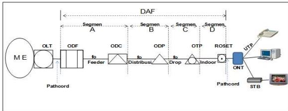
GAMBAR 1 ARSITEKTUR JARINGAN FTTH
