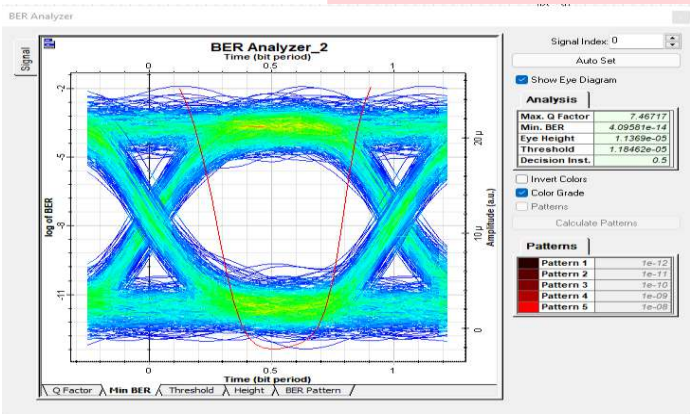
GAMBAR 11 HASIL SIMULASI BER
