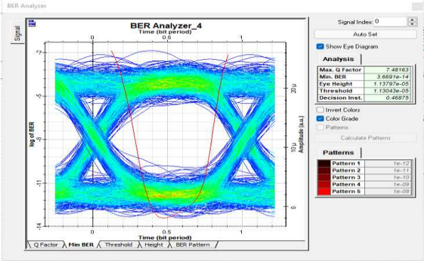
GAMBAR 10 HASIL SIMULASI BER
