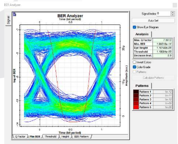
GAMBAR 11 HASIL SIMULASI BER
