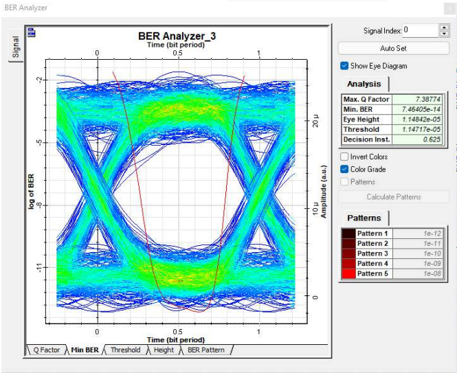
GAMBAR 12 HASIL SIMULASI BER
