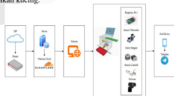
GAMBAR 1. DESAIN SISTEM
