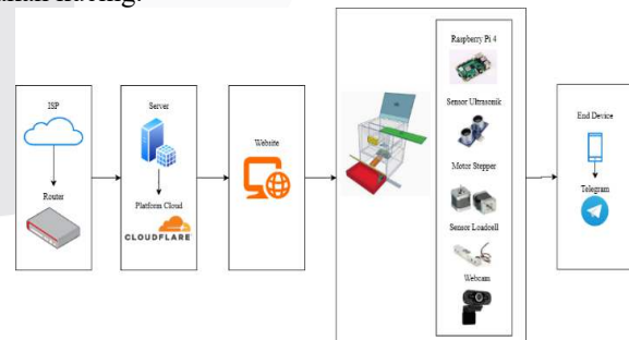
GAMBAR 1. DESAIN SISTEM
