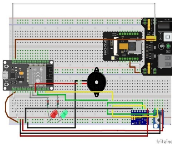
GAMBAR 4. DESAIN PERANGKAT KERAS
