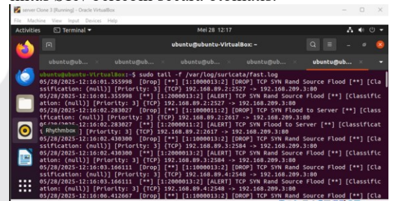
Gambar 15 menampilkan fast.log dari suricata yang dijalankan selama pengujian serangan SYN Flood . Dari tampilan log terlihat bahwa suricata berhasil mendeteksi pola serangan TCP SYN Rand Source Flood yang berasal dari IP attacker 192.168.89.2 dan 192.168.89.3, dengan target server 192.168.209.3 pada port 80. Setiap entri log menunjukkan bahwa paket-paket tersebut tidak hanya dikenali sebagai serangan, tetapi juga secara aktif diblokir, ditandai dengan label [Drop] . Suricata mencatat dan memberikan informasi jenis ancaman melalui label seperti " TCP SYN Flood to Server " dan " TCP SYN Rand Source Flood ".
