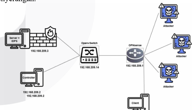
GAMBAR 3 (TOPOLOGI JARINGAN)
