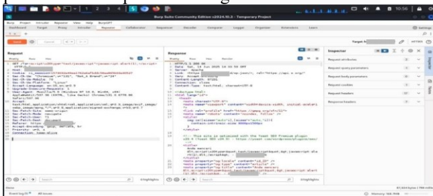
GAMBAR 10 PENGUJIAN DARI BURP SUITE
