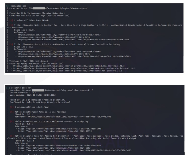
GAMBAR 9 HASIL DARI WPSCAN
