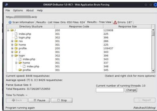
GAMBAR 19 Hasil Pengujian DirBuster
