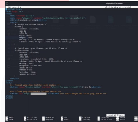
GAMBAR 12 Skrip Pengujian Clickjacking
