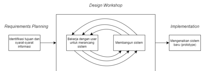
GAMBAR 2 Ilustrasi Model RAD
