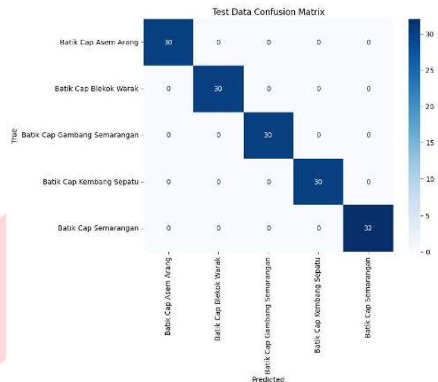
GAMBAR 8 (CONFUSION MATRIX)
