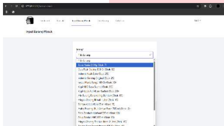
GAMBAR 17 (PILIH BARANG)
