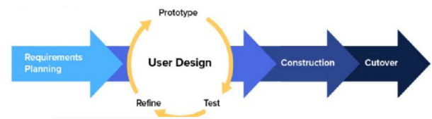
GAMBAR 1 (METODE RAD)
