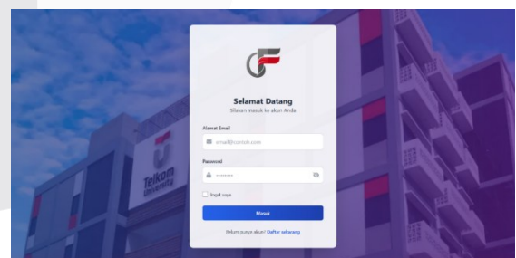
GAMBAR 16 (HALAMAN LOGIN)
