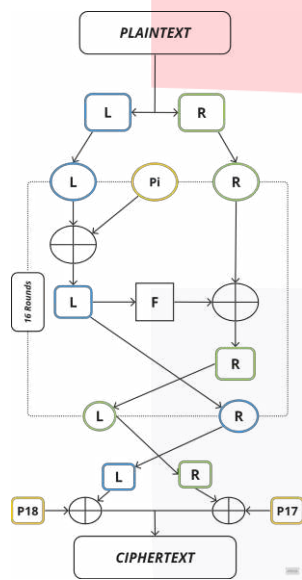
GAMBAR 5 (SKEMA ALUR ALGORITMA BLOWFISH)
