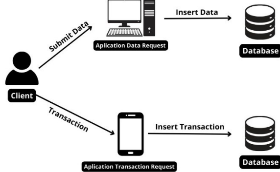
GAMBAR 1 (ILUSTRASI DATABASE)
