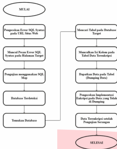
GAMBAR 11 (ALUR SKEMA PENGUJIAN SISTEM)
