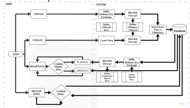
GAMBAR 6 ARSITEKTUR SISTEM
