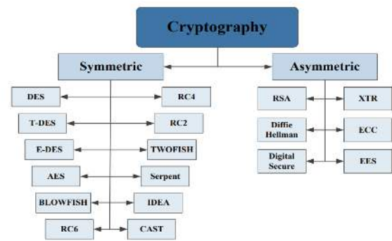
GAMBAR 2 (KLASIFIKASI KRIPTOGRAFI)
