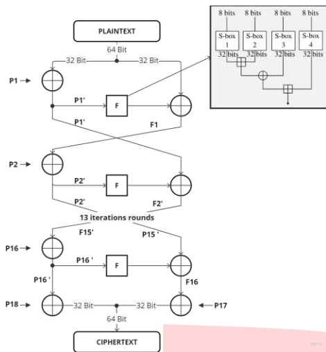
GAMBAR 4 (DIAGRAM ALUR ENKRIPSI ALGORITMA BLOWFISH)
