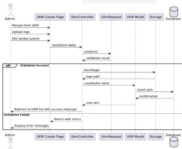
Gambar 4. Contoh Sequence Diagram Admin Membuat UKM
