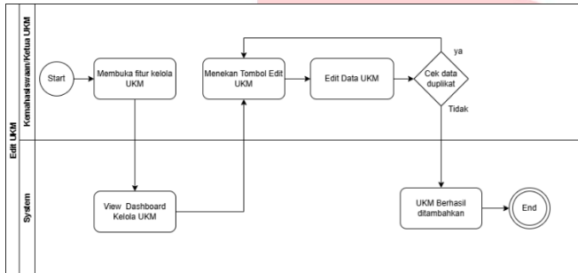
Gambar 3. Contoh Activity Diagram Admin/Ketua UKM Melakukan Edit UKM
