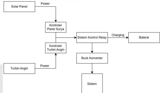
GAMBAR 2 (DESAIN SISTEM)
