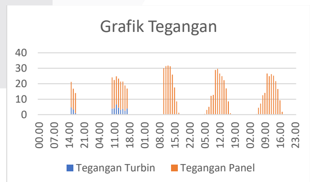
GAMBAR 5 (GRAFIK TEGANGAN)
