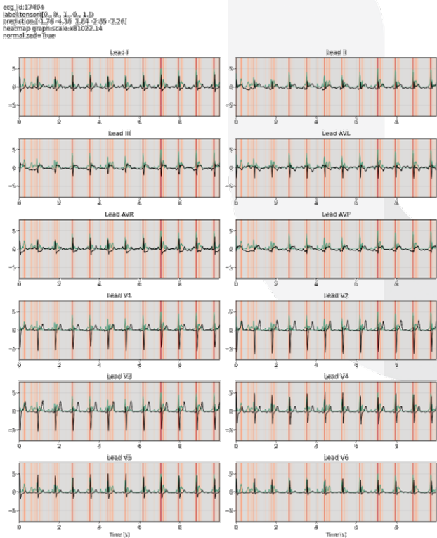
GAMBAR 3 Sampel Grad-CAM pada InceptionTime, kasus true positive MI
