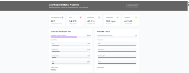
GAMBAR 4 Tampilan Utama
