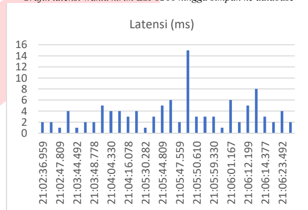
GAMBAR 6 Grafik latensi waktu kirim ESP8266 hingga simpan ke database
