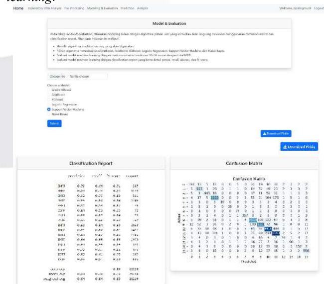
GAMBAR 12 Tahap dan Hasil Modeling dan Evaluation
