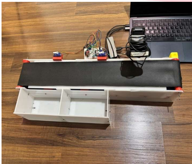
GAMBAR 12 (Gambar fisik prototipe system)
