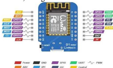
GAMBAR 2 (NodeMCU ESP8266)
