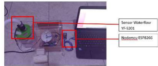
GAMBAR 4 Pengujian Sensor YF-S201
