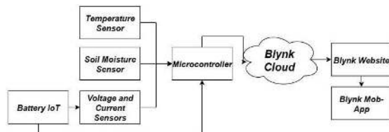
GAMBAR 1 Blok diagram sistem IoT.
