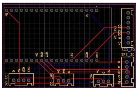
GAMBAR 3 Desain PCB
