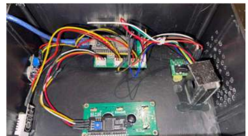
GAMBAR 4 Tampilan Bagian Dalam Rangkaian
