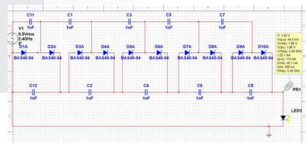
(b) Frekuensi 2,4 GHz GAMBAR 18 Rangkaian rectifier
