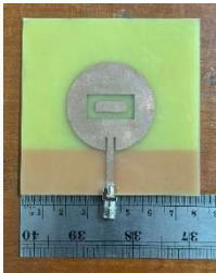
GAMBAR 9 Fabrikasi antenna mikrostrip tampak depan
