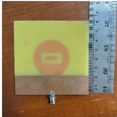
GAMBAR 10 Fabrikasi antenna mikrostrip tampak belakang
