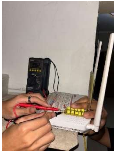
GAMBAR 21 Pengujian rectenna 2
