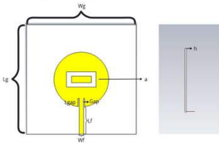
GAMBAR 7 Desain antenna mikrostrip tampak depan dan samping
