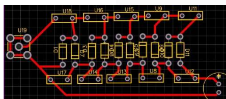
GAMBAR 5 Desain PCB rectifier 2
