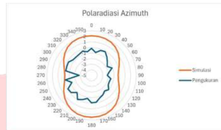
GAMBAR 16 Pola radiasi azimuth 2,4 GHz
