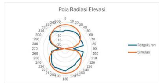
GAMBAR 15 Pola radiasi elevasi 1,8 GHz
