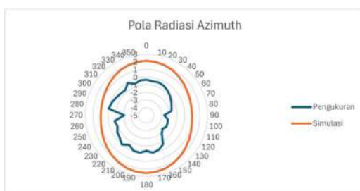
GAMBAR 14 Pola radiasi azimuth 1,8 GHz
