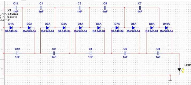
GAMBAR 3 Skematik rangkaian rectifier
