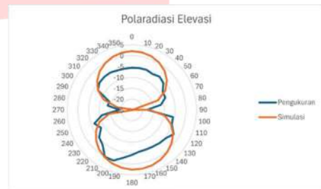
GAMBAR 17 Pola radiasi elevasi 2,4 GHz
