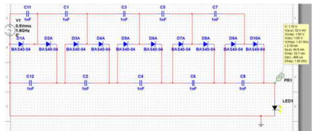
GAMBAR 11 (Hasil simulasi frekuensi 1,8 GHz)
