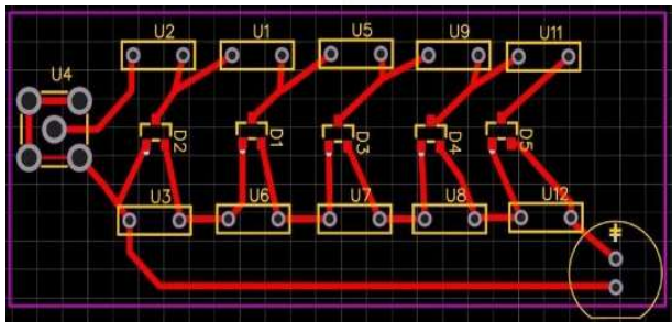
GAMBAR 9 (Desain PCB rectifier 1)
