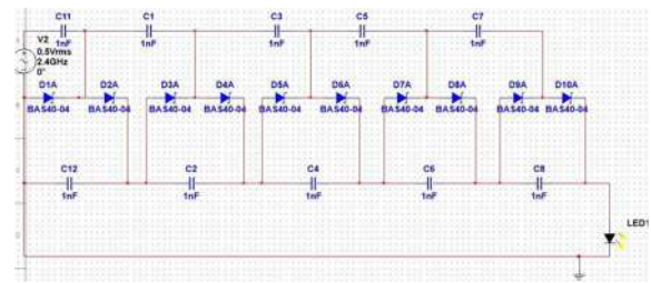
GAMBAR 5 (Skematik rangkaian rectifier)
