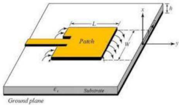
GAMBAR 1 (Antena Mikrostrip)
