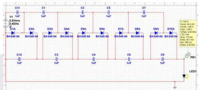
GAMBAR 12 (Hasil simulasi frekuensi 2,4 GHz)
