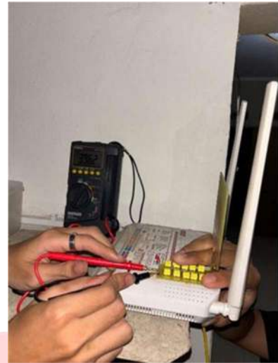
GAMBAR 15 (Pengujian Rectenna dengan Wi-Fi)
