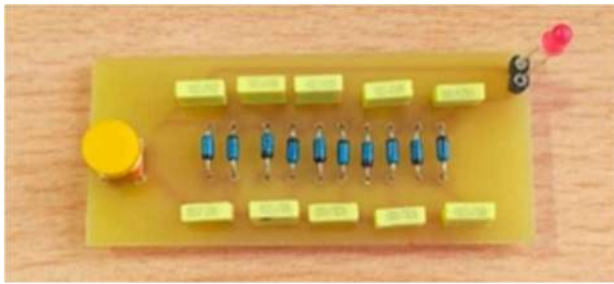
GAMBAR 7 (Tampak depan rectifier dengan dioda 1N5711)
