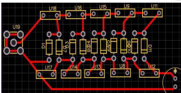
GAMBAR 10 (Desain PCB rectifier 2)
