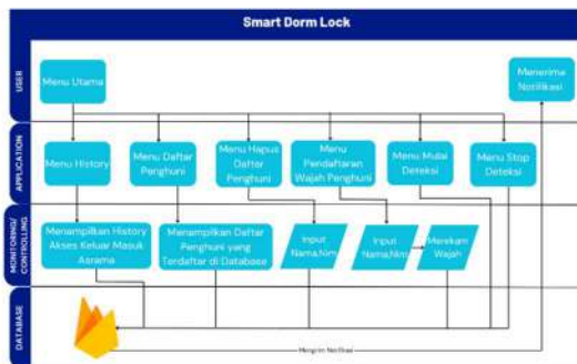
GAMBAR 1 Arsitektur Sistem
