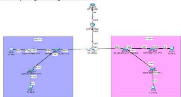
GAMBAR 2 Topologi Jaringan
