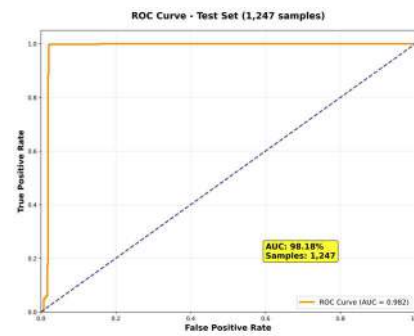
GAMBAR 5 Kurva ROC
