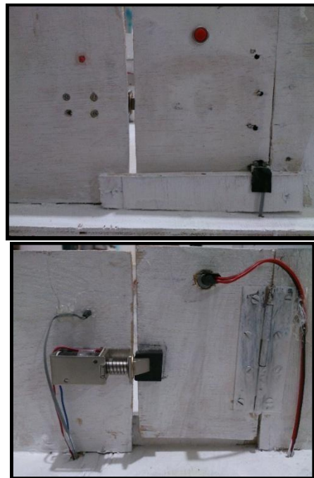
Gambar 4.2 Tampak Depan dan Belakang SLD,PB, dan Limit Switch
