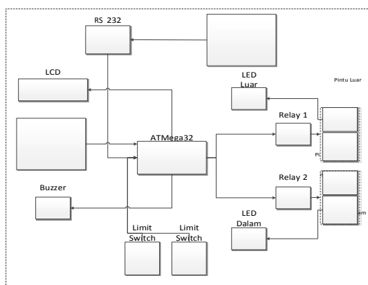
Gambar 3.1 Miniatur Sistem Pusat
