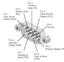
Gambar 2.7 Spesifikasi Pin pada RS – 232 DB 9
