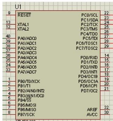
Gambar 4.3 Port dan Pin pada ATmega32
