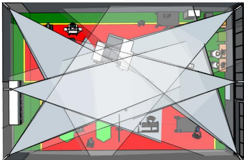
Gambar 2 Visualisasi Jangkauan Area CCTV
