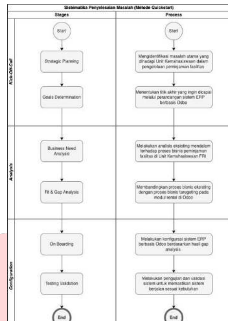
Gambar III. 2 Sistematika Penyelesaian Masalah
