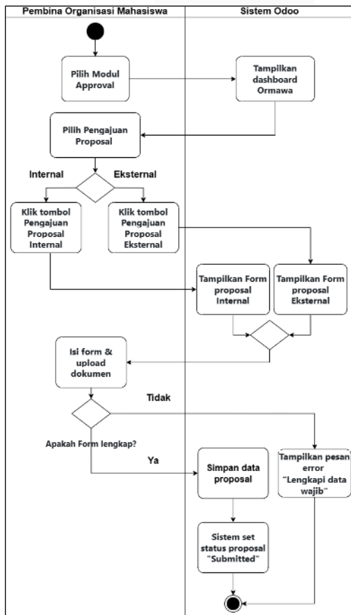
GAMBAR 10 (Activity Diagram Mengajukan Proposal Kegiatan)
