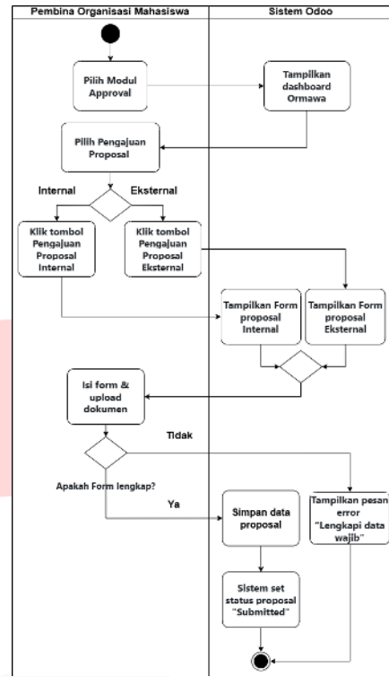
GAMBAR 11 (Activity Diagram Mengajukan Pendanaan)
