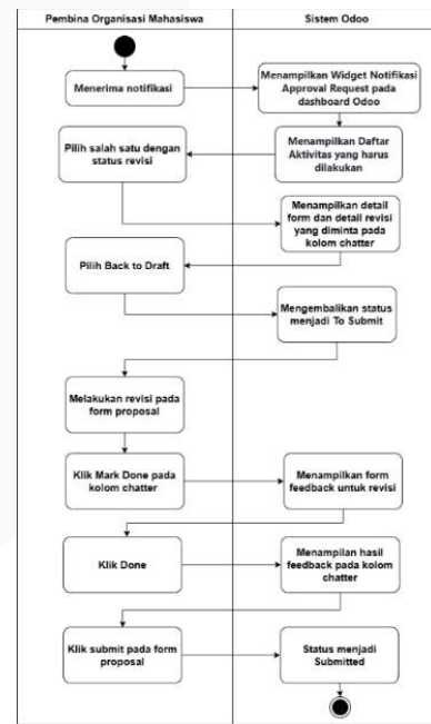
GAMBAR 12 (Activity Diagram Melakukan Revisi Proposal)
