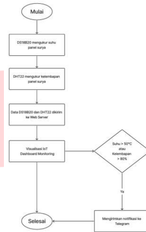
Gambar 2 Monitoring Suhu dan Kelembapan Panel Surya
