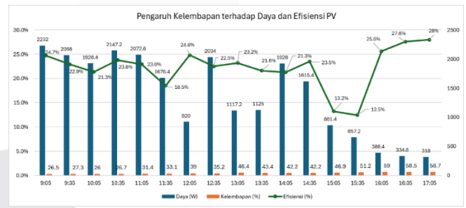
Gambar 8 Pengaruh Kelembapan lingkungan terhadap Daya dan Efisiensi
