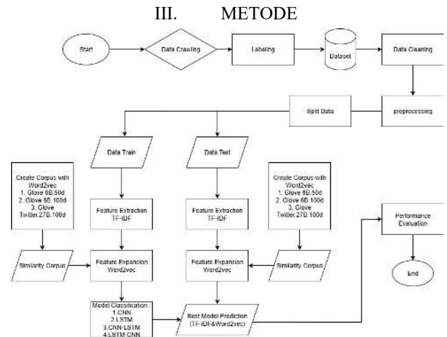
GAMBAR 1 Sistem Deteksi Bunuh Diri
