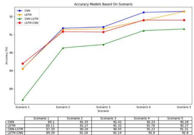
GAMBAR 3 Peningkatan akurasi semua skenario
