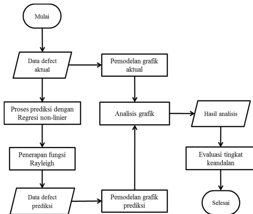
Gambar 2. Arsitektur sistem
