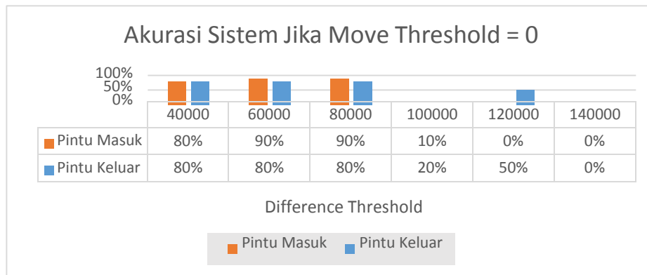
Gambar 2. Grafik Akurasi Sistem Jika Move threshold = 0
