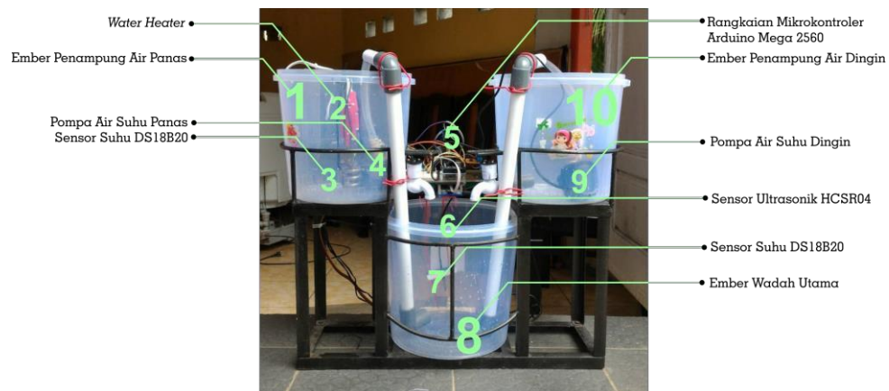
Gambar 7. Perancangan alat keseluruhan
