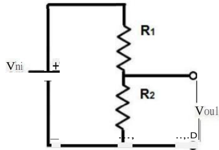
Gambar 4. Sensor Tegangan
