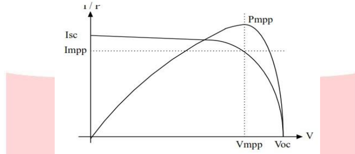
Gambar 1. Karakteristik untuk solar cell, Current vs Voltage (I-V) and current vs power (I-P)
