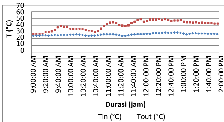
Gambar 4.8 Grafik Temperatur terhadap Waktu pada Debit 0.3 liter/menit
