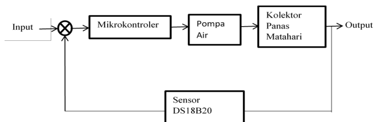
Gambar 3.4 Blok Diagram Sistem Penelitian Kolektor Plat Datar
