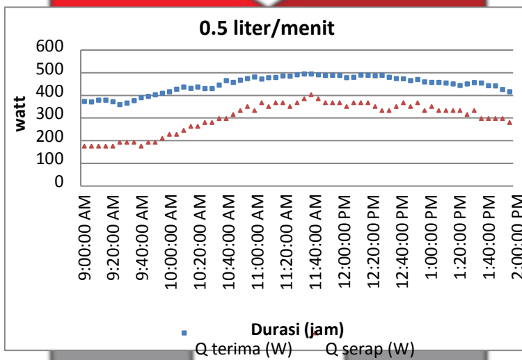
Gambar 4.5 Grafik Perbandingan (Q terima) terhadap (Q serap)
