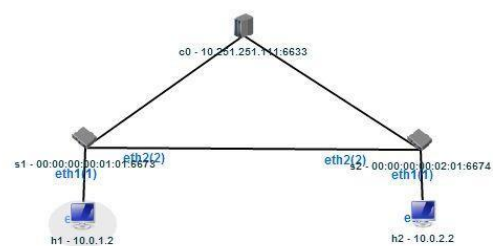
Gambar 2.5.7.a Topologi 2 switch
