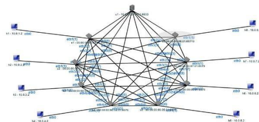
Gambar 2.5.7.c Topologi 8 switch
