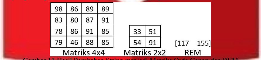
Gambar 11 Hasil Perubahan String menjadi Matriks Orde Genap dan REM
