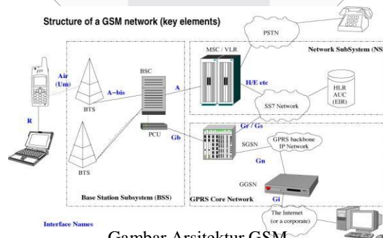
Gambar Arsitektur GSM
