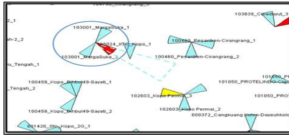
Gambar Adjacent Interference BTS Margasuka_2 dengan BTS Kopo Permai_3
