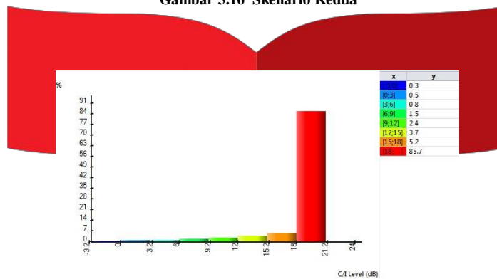
Gambar 3.17 Histogram C/I Skenario Kedua
