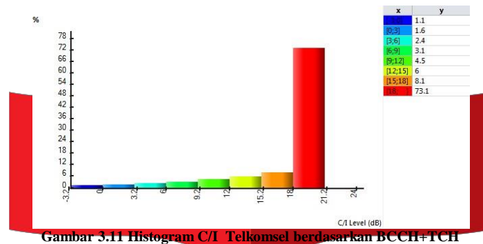
Gambar 3.11 Histogram C/I Telkomsel berdasarkan BCCH+TCH
