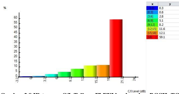
Gambar 3.8 Histogram C/I Telkom FLEXI berdasarkan BCCH+TCH
