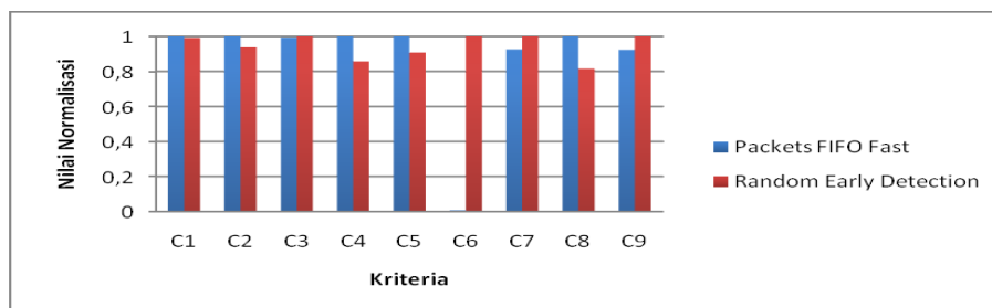
Gambar 5. Perbandingan Hasil Pengukuran Antara PFIFO Fast dengan RED pada kondisi Static ad-hoc network dengan receiver bergerak.
