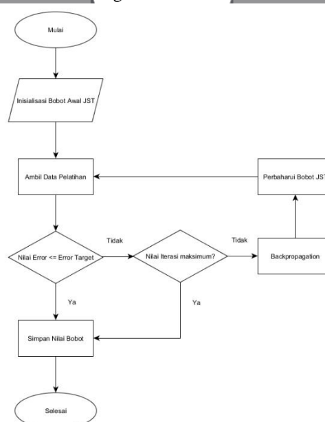
Gambar 2. Flowchart Pelatihan JST
